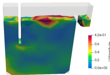
Figura 8. Simulación del tanque sedimentador secundario.
